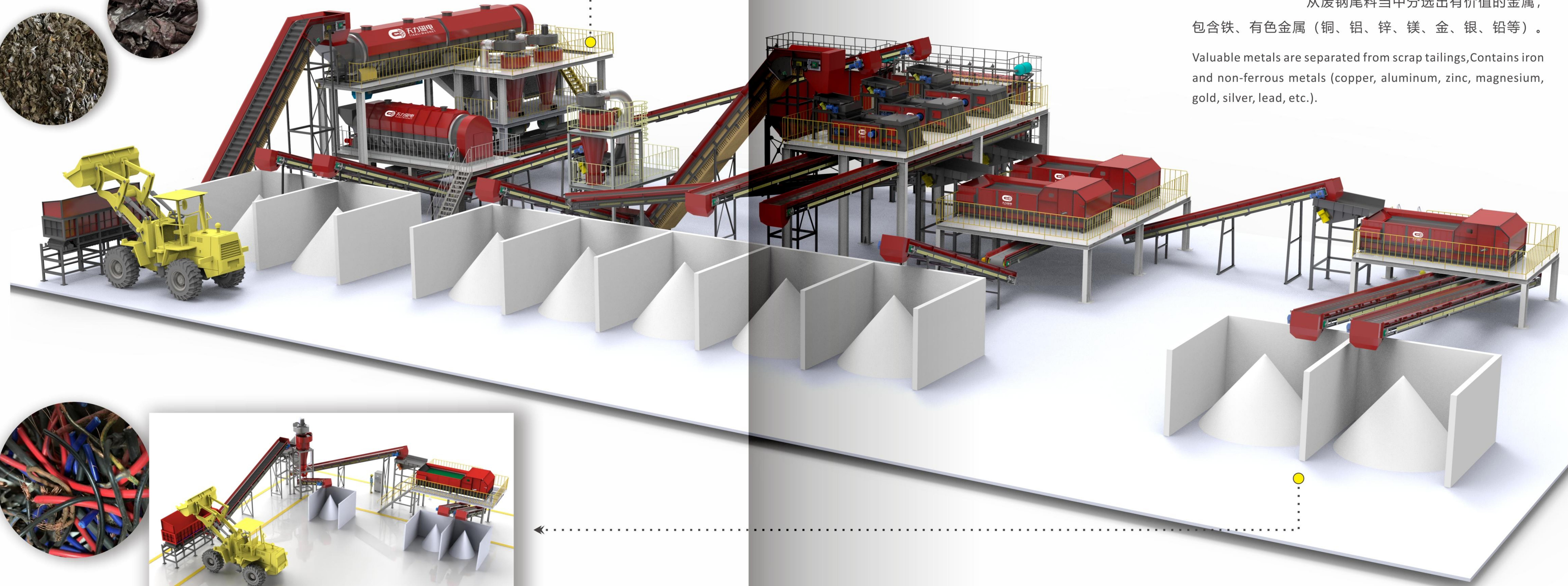
不锈钢分选系统方案
